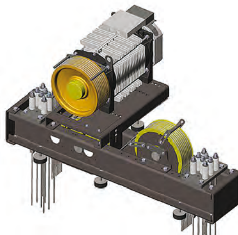
Fot. 6 Wyciągarka MRL, nowoczesne urządzenie windy, które łączy dużą moc z małymi wymiarami. Global Lift
